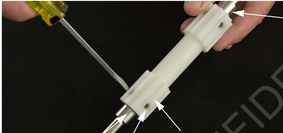
Eje impulsado Tornillos de sujeción Extremo de la rueda dentada
