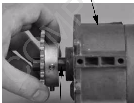
Chaveta del eje del motorreductor
