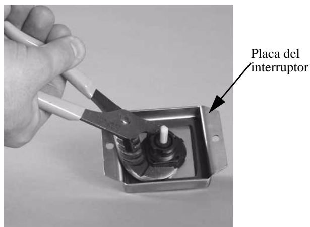
Anillo de bloqueo
