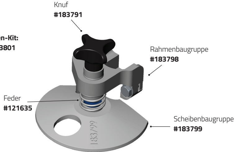
Schnitttiefenscheiben-Kit: X1850 #184479
